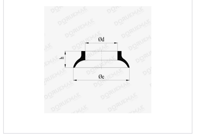
FIG. 02 Teknik resim
