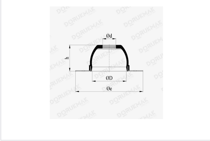
FIG. 01 Teknik resim
