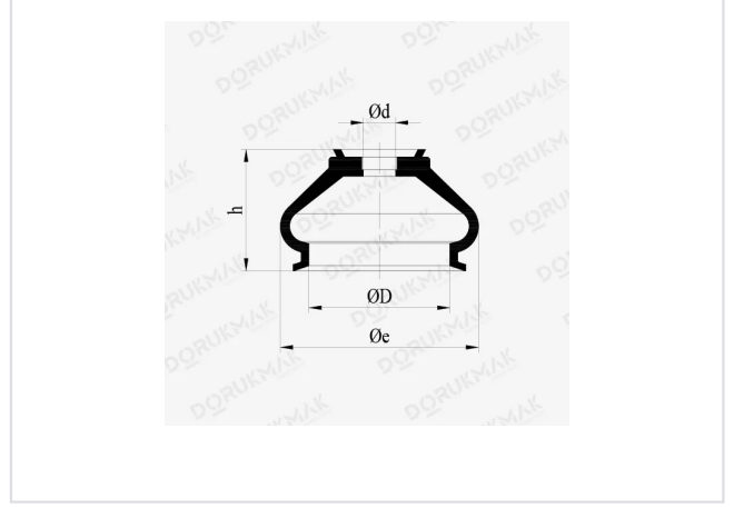
FIG. 02 Teknik resim
